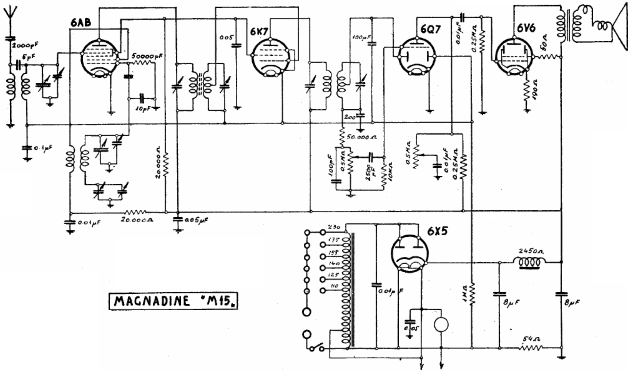
68. — MAGNADYNE RADIO. — Mod. « M 15 » Serie normale. — Produzione 1939-1940. — Media frequenza: 471 kHz. Valvole Balilla. — (Stesso schema anche per il mod. KENNEDY 415 K).
